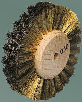
ZBL80 Brosse circulaire laiton 4 rangs Ø 80
